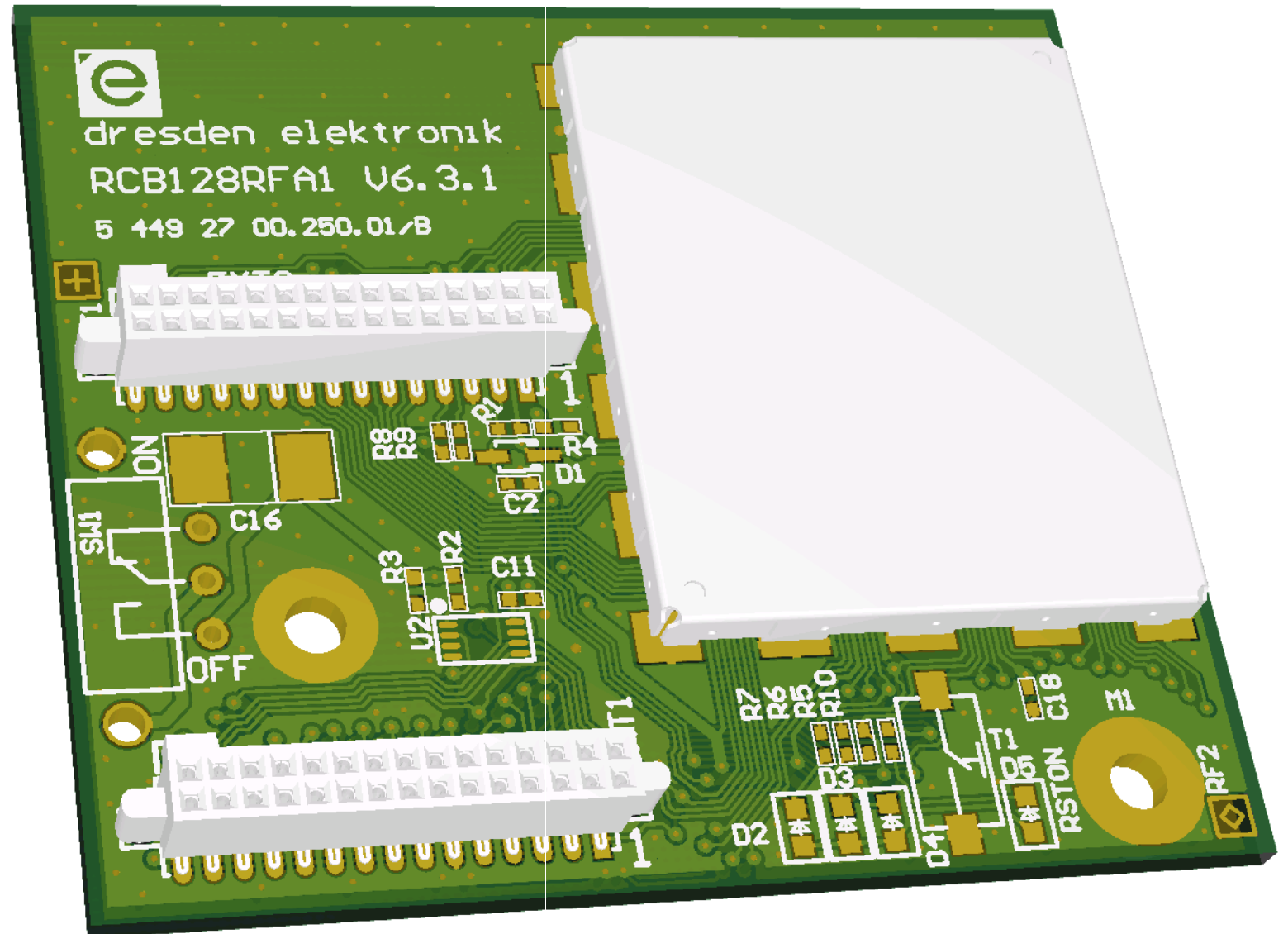
RCB128RFA1_V6.3.1 LP-B 5 449 27 00.200.01 BL1(3)
